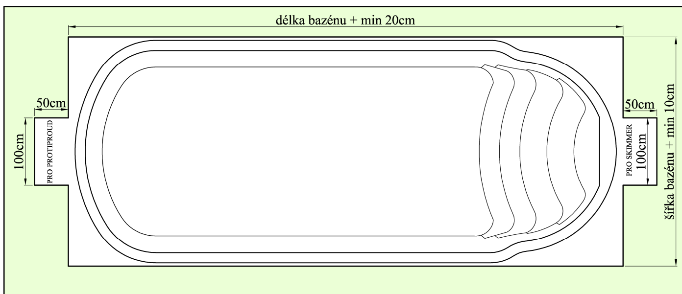
půdorys výkopu
