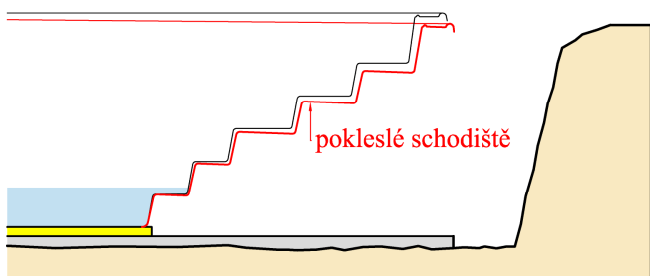
v případě pokleslého schodiště je nutné toto vyrovnat pomocí podepření
