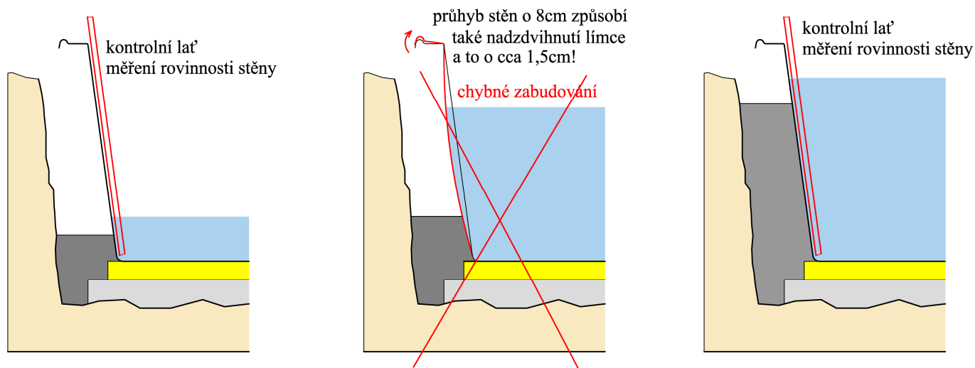
kontrola rovinnosti stěn ve svislém směru
