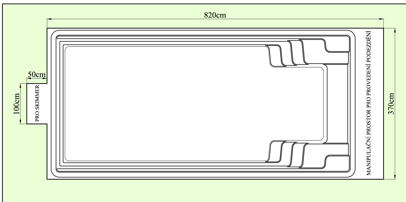
půdorys výkopu
